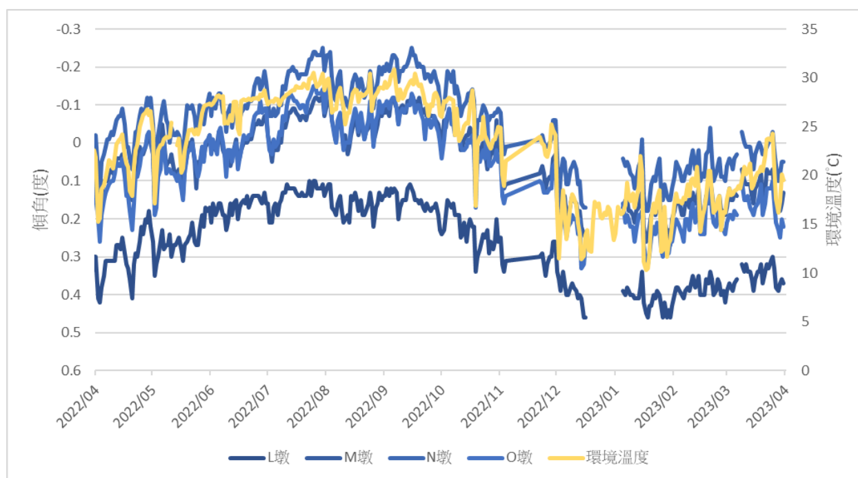
圖 5 南灣湖樁柱傾角與環境溫度變化趨勢（2022 年 4 月~2023 年 3 月）
