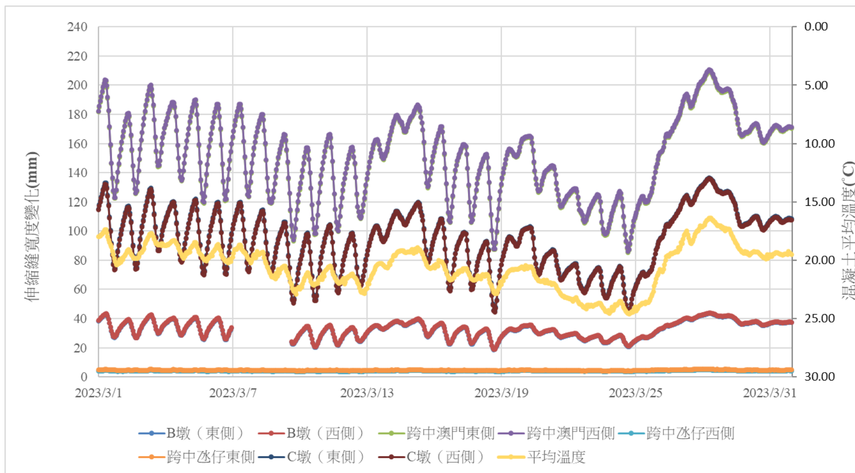
圖 3 伸縮縫寬度變化圖 (2023 年 3 月)
