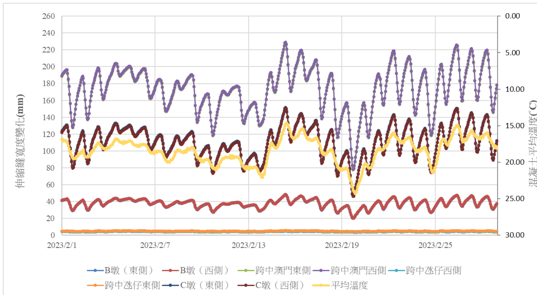
圖 2 伸縮縫寬度變化圖（2023 年 2 月）
