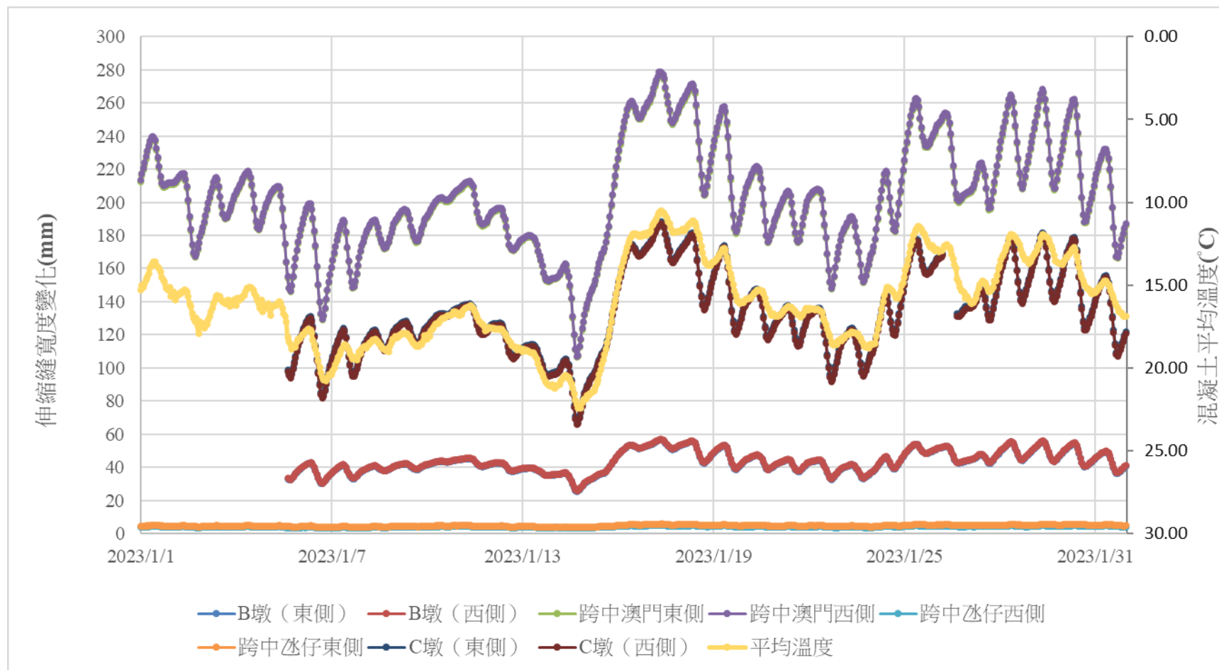
圖 1 伸縮縫寬度變化圖（2023 年 1 月）
