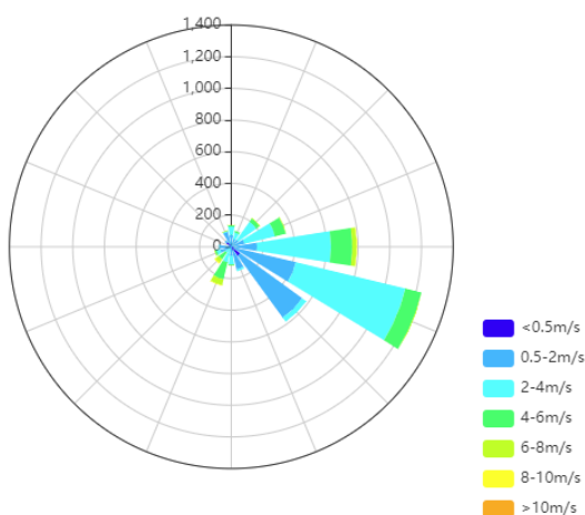
圖 8 2023 年 3 月十分鐘風玫瑰圖
