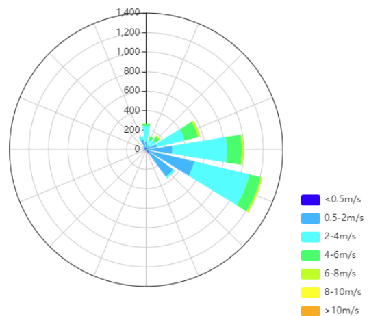
圖 7 2023 年 2 月十分鐘風玫瑰圖
