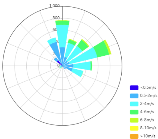
圖 6 2023 年 1 月十分鐘風玫瑰圖
