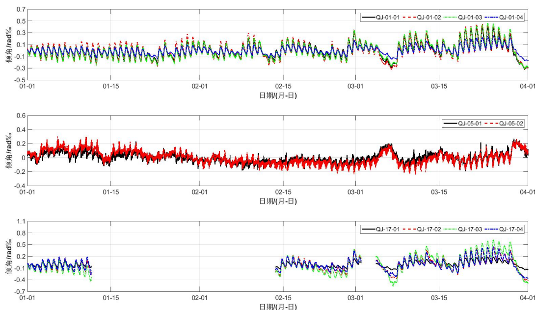
圖 5-2 傾角時程圖
