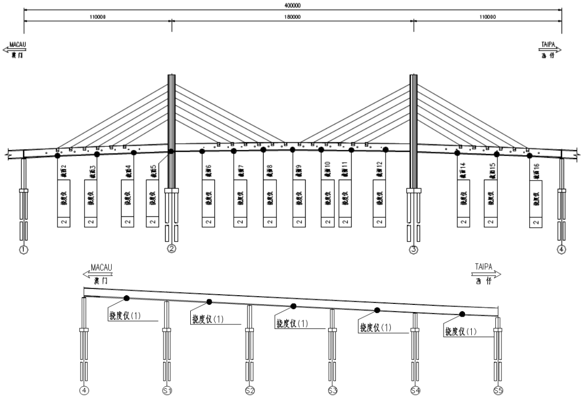
圖 6-1 主樑豎向撓度監測點佈置圖
