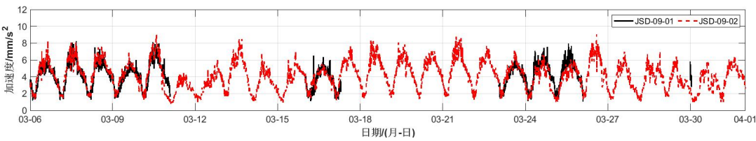
圖 9-3 加速度 RMS 時程圖
