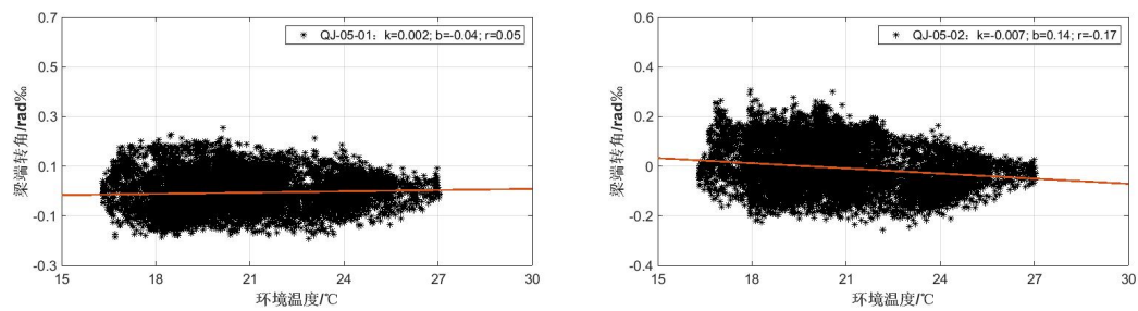
圖 5-3 傾角同結構溫度相關性分析
