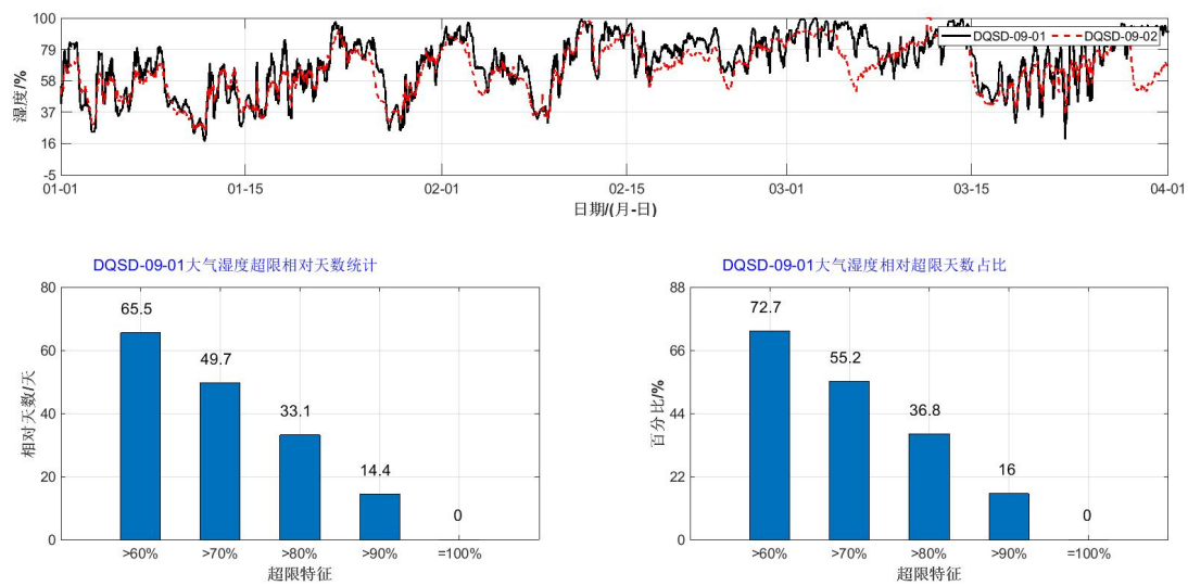
圖 3-4 箱梁內部大氣相對濕度趨勢圖
