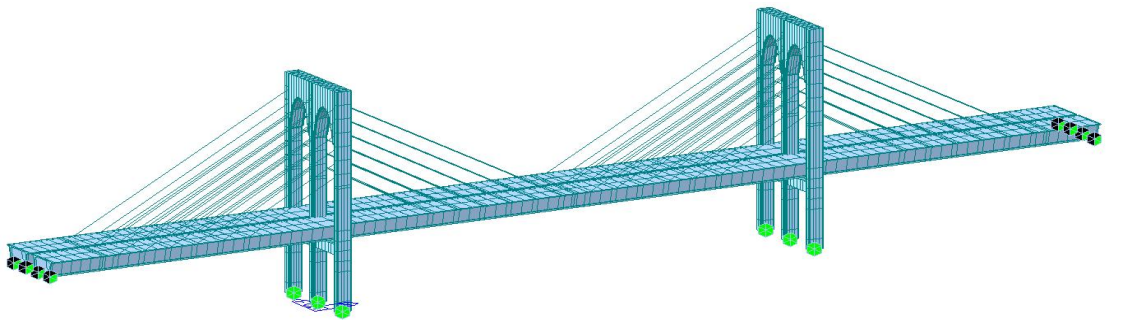
圖 8-2 結構縱向計算總體模型
