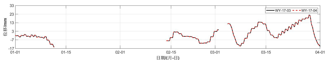
圖 5-5 支座位移季度相對變化趨勢
