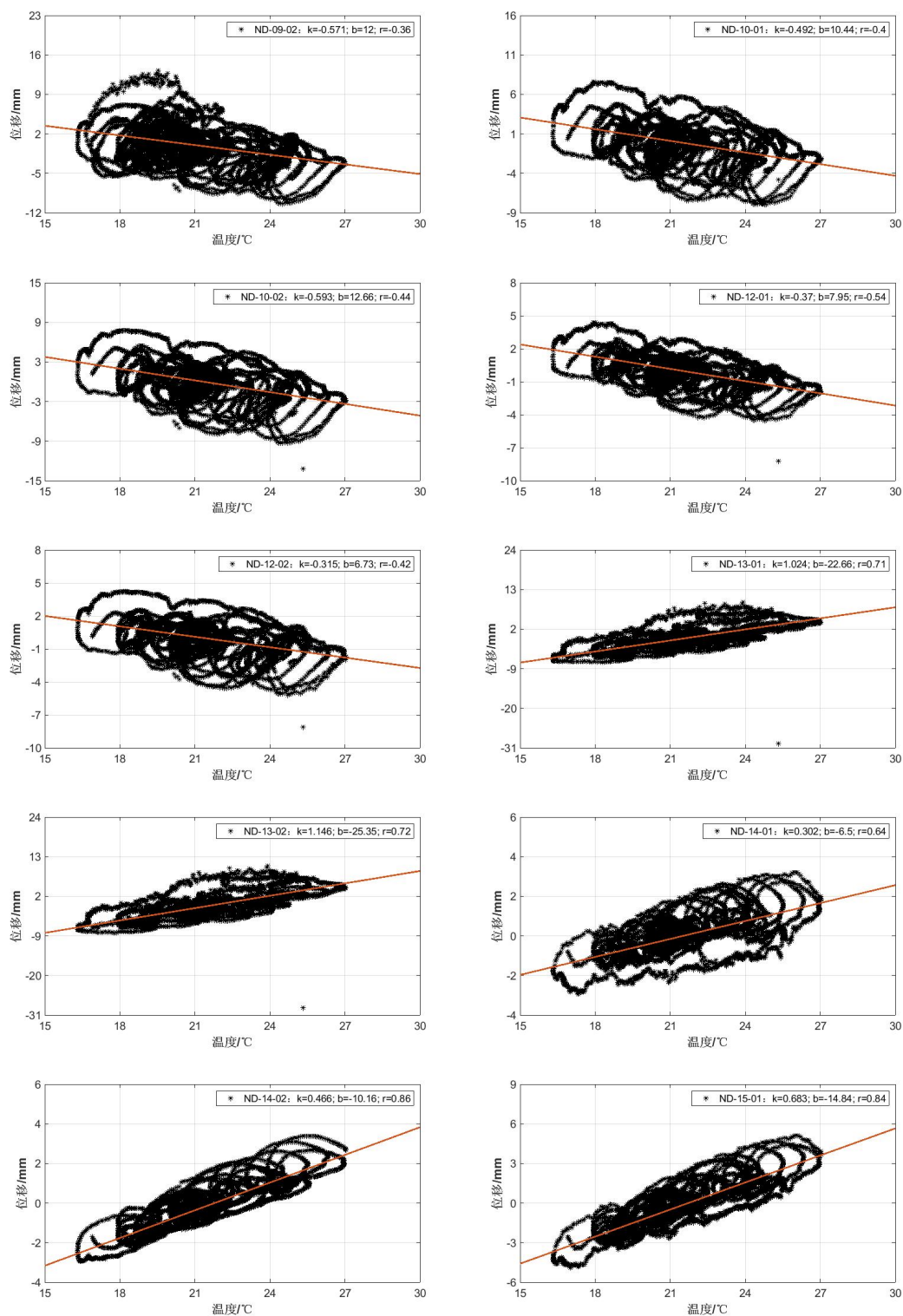
圖 6-5 溫度作用引起樑體變形相關性
