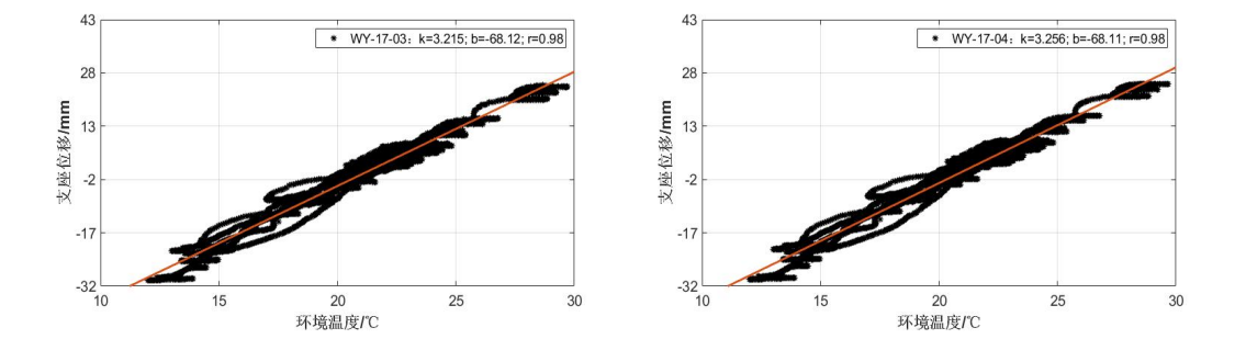
圖 5-6 支座位移同大氣溫度相關性分析
