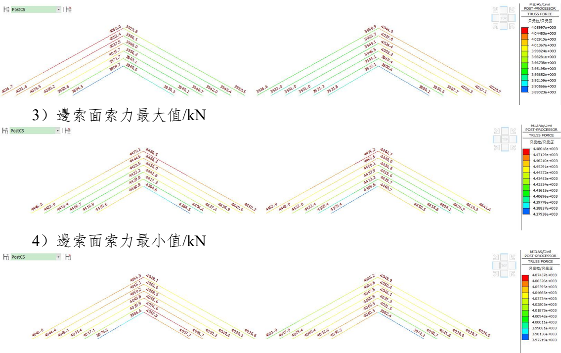
图 8-3 运营阶段斜拉索索力图/kN
